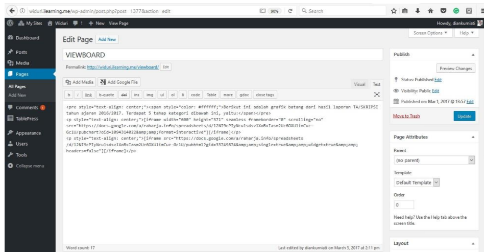
Gambar 8. Page Widuri
